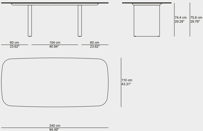
DINING TABLE - 240X110CM 03252-XX-XX
